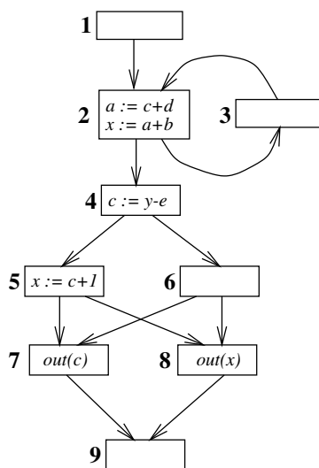
Abb. 1. Ausgangsprogramm als knotenbenannter BB-Flußgraph.
