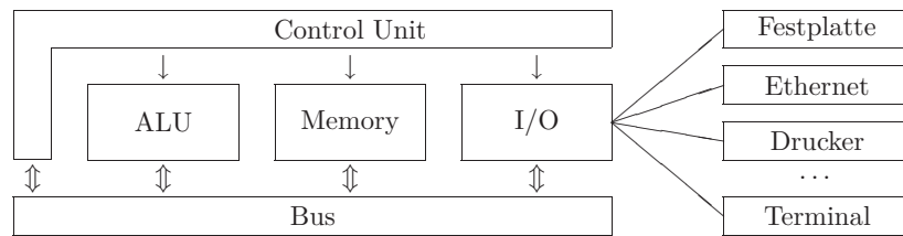
Abbildung 1.12: Von Neumann-Architektur
