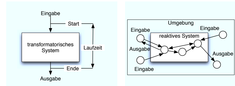
Abbildung 2.50: Links ein transformatorisches System, rechts ein reaktives
