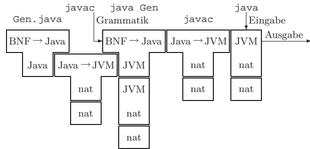
Abbildung 1.18: Beispiel zur kombinierten Verwendung mehrerer Compiler
