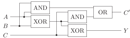
Abbildung 1.10: Volladdierer bestehend aus mehreren Gattern
