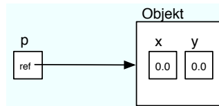
Abbildung 3.3: Variable p enthält Referenz auf Objekt vom Typ Punkt
