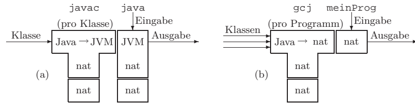
Abbildung 1.17: Vom Code zur Ausführung (a) mit und (b) ohne Zwischencode
