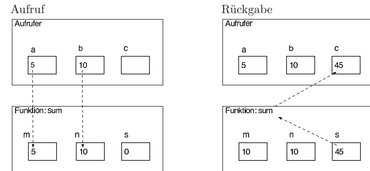
Abbildung 2.44: Aufruf der Pascal-Funktion sum mit call-by-value -Schnittstelle. Parameterübergaben beim Funktionsaufruf sind als gestrichelte Pfeile dargestellt. Werte der formalen Parameter ändern sich während der Berechnung. Für den Aufrufer sind diese Änderungen ohne Auswirkungen. Bei der Rückkehr aus der Funktion wird der Wert 45 geliefert und an c zugewiesen.
