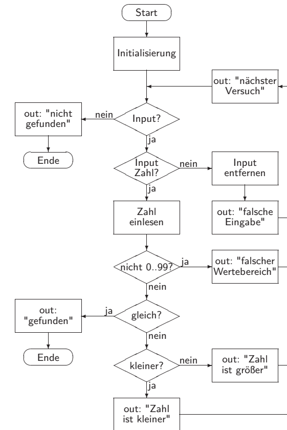
Abbildung 1.20: Flussdiagramm zur Darstellung des Programmablaufs
