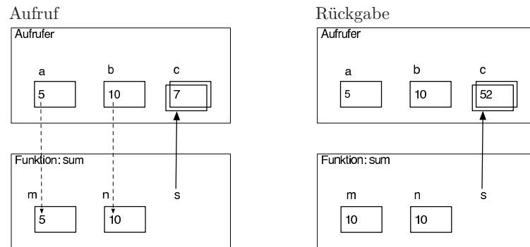
Abbildung 2.46: Aufruf der Pascal-Prozedur addsum mit call-by-reference -Schnittstelle. s ist ein Variablenparameter , während m und n Wertparameter sind. Implizite Zuweisungen beim Aufruf sind als gestrichelte Pfeile dargestellt. Der durchgehende Pfeil veranschaulicht, dass über s in der Prozedur dieselbe Variable angesprochen wird wie über c im Aufrufer.
