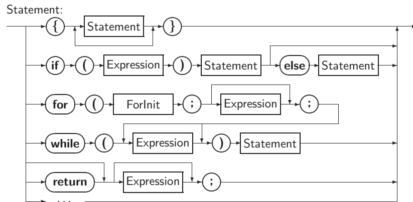
Abbildung 1.16: Veranschaulichung der Grammatikregel aus Abbildung 1.15
