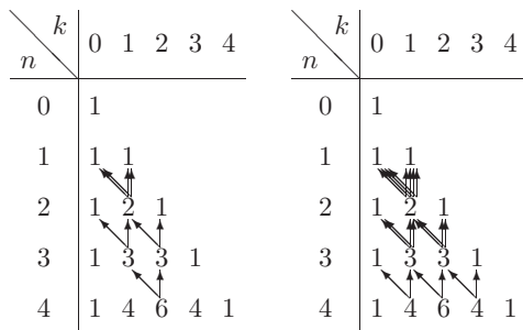
Abbildung 2.40: Links: Beim Aufruf von \text{binom}(4,2) kommt es zu weiteren rekursiven Aufrufen, wobei \text{binom}(2,1) und folglich \text{binom}(1,1) und \text{binom}(1,0) je zweimal berechnet wird. Die Anzahl der Aufrufe wächst mit n . So kommt es beim Aufruf \text{binom}(6,3) (nicht eingezeichnet) bereits je 4 mal zum Aufruf \text{binom}(2,1) . Rechts: Bei der Berechnung der 5. Zeile gibt es 22 rekursive Aufrufe.
