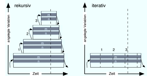
Abbildung 2.32: Die während der Ausführung von int ggt(int, int) vorhandenen lokalen Variablen, links in der rekursiven und rechts in der iterativen Variante. Jede Methodenausführung hat ihren eigenen Speicherbereich. Die Speicherbereiche aufgerufener Methoden liegen oberhalb jener der aufrufenden Methoden (siehe Aufrufpfeile). Für jeden rekursiven Aufruf werden weitere Variablen angelegt. Die iterative Variante kommt dagegen mit einer einzigen Methodenausführung und daher weniger Variablen aus.
