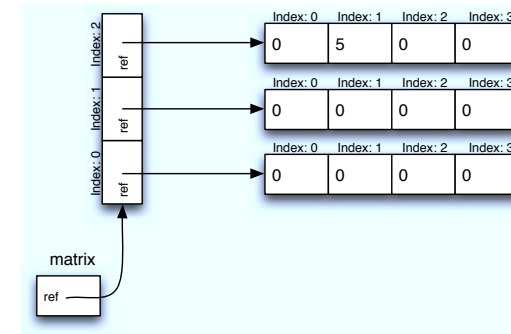
Abbildung 2.36: Mehrdimensionales Array
