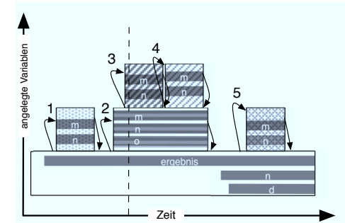
Abbildung 2.30: Speicherbereiche der Methodenausführungen entsprechend Listing 2.28. Die Bereiche aufgerufener Methoden liegen oberhalb jener der aufrufenden Methoden, siehe Aufruffeile. Nach Aufruf 3 (gestrichelte Linie) sind nur die zwei Variablen der obersten Methode zugreifbar. Die aufrufenden Methoden sind unterbrochen, bis die aufgerufenen Methoden fertig sind.
