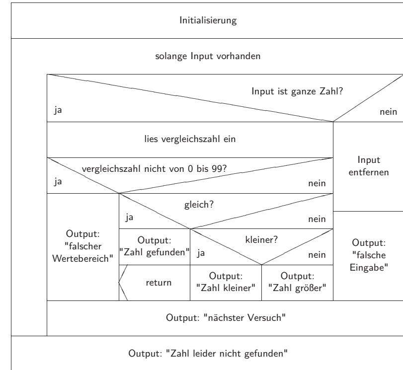
Abbildung 1.21: Struktogramm zur Darstellung des Programmablaufs
