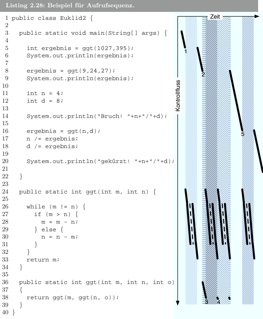
Abbildung 2.29: Ausführungsreihenfolge (grafisch)
