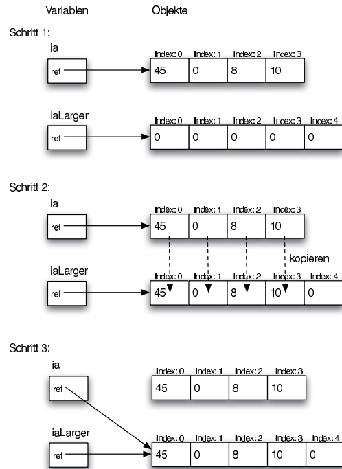
Abbildung 2.35: Veranschaulichung der Schritte entsprechend Listing 2.34
